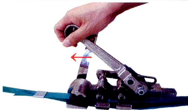
②引き締めレバーを前方に倒し、周回させたバンドをセットします シールはあらかじめ通しておきます
