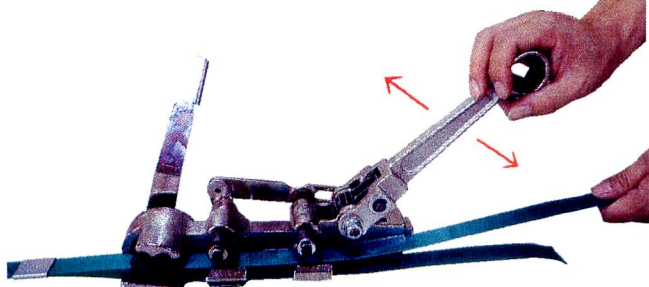
③引き締めレバーを前後に操作し引き締め ラックが移動しない為その場で無限引き締め可能
