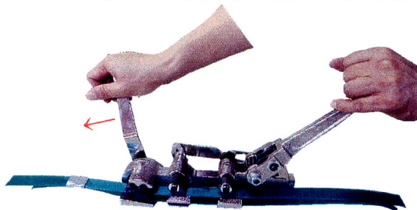
⑤カッターレバーを前方に倒しバンドを切断 独自の構造により t 0.7 の帯鉄も楽々切断可能
