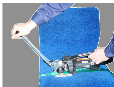
⑥引締レバーを前方に 操作すると
