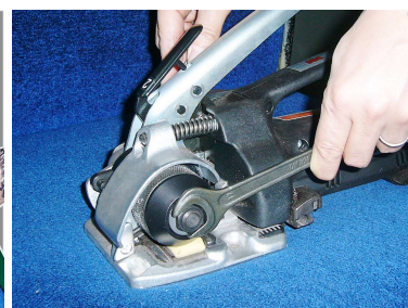
★トルクリミッター 引締力のMAX値調整
