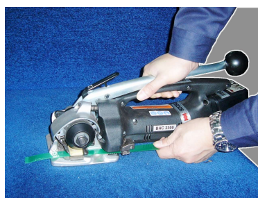
②引締レバーを押しながら バンド先端をセットします
